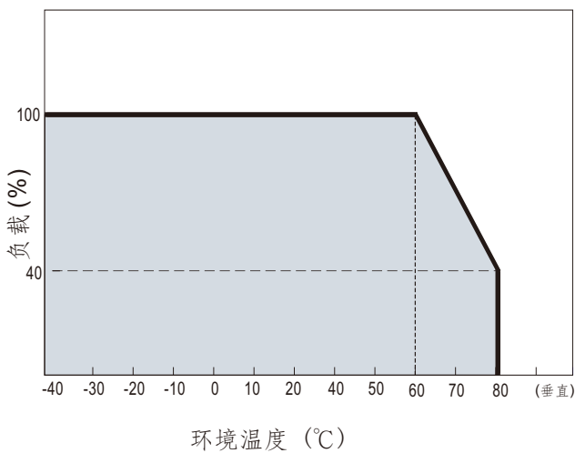
■ 减额曲线
