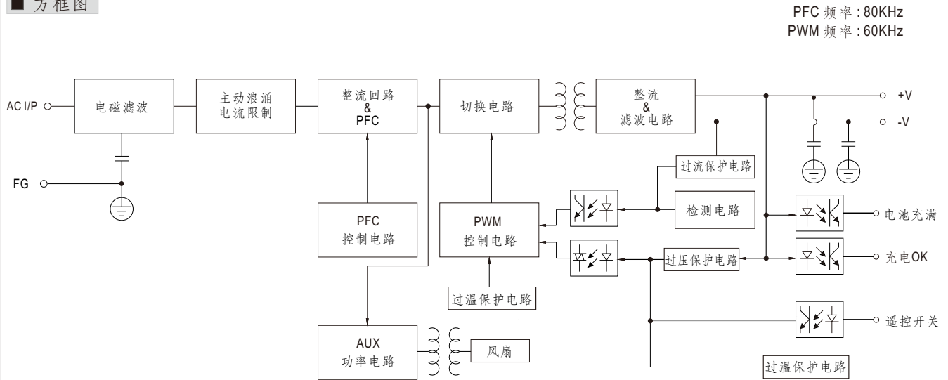
■ 方框图
